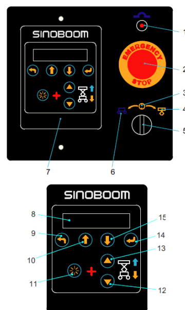
Figura 6-1 Modulo comandi a terra
