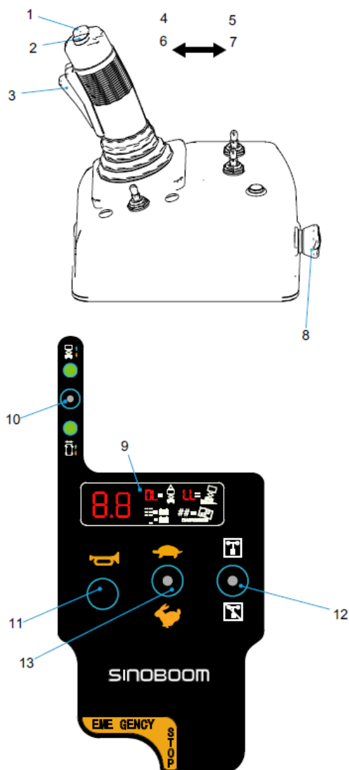
Figura 6-2 Modulo comandi sulla piattaforma (SINOBOOM)
